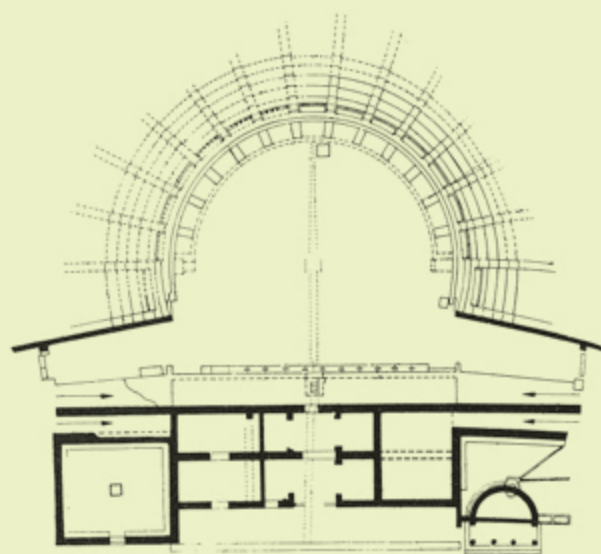
Εικ. 3 Κάτοψη του θεάτρου.
